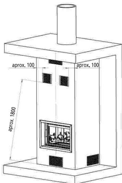
Figura nº7 - Esquema exterior del cerramiento
