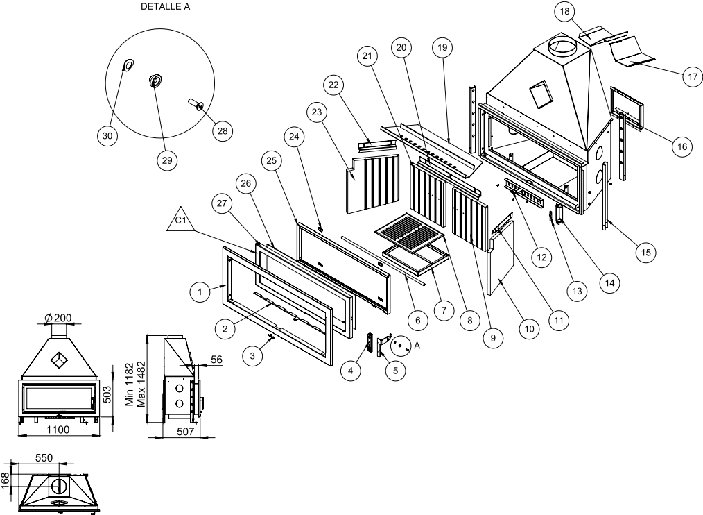
DETALLE A
