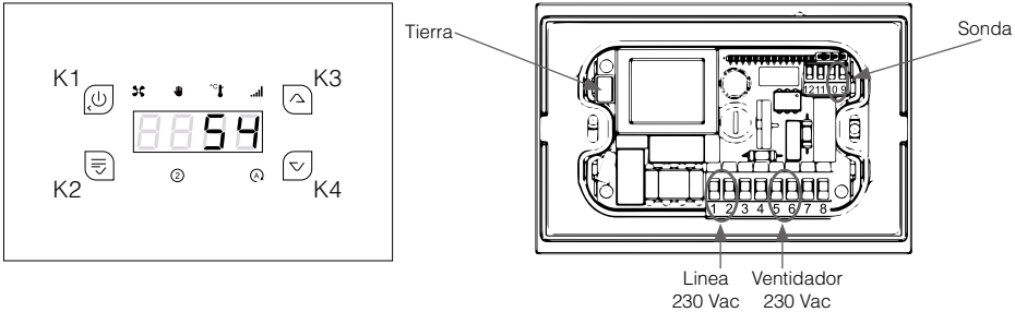
Aspecto externo y conexiones eléctricas
