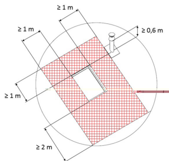
A - B Okno dachowe
