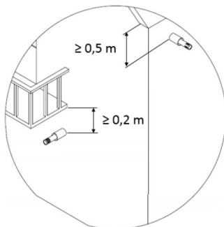
D - E Ogiegłość poniżej balkonu i od krawędzi dachu
