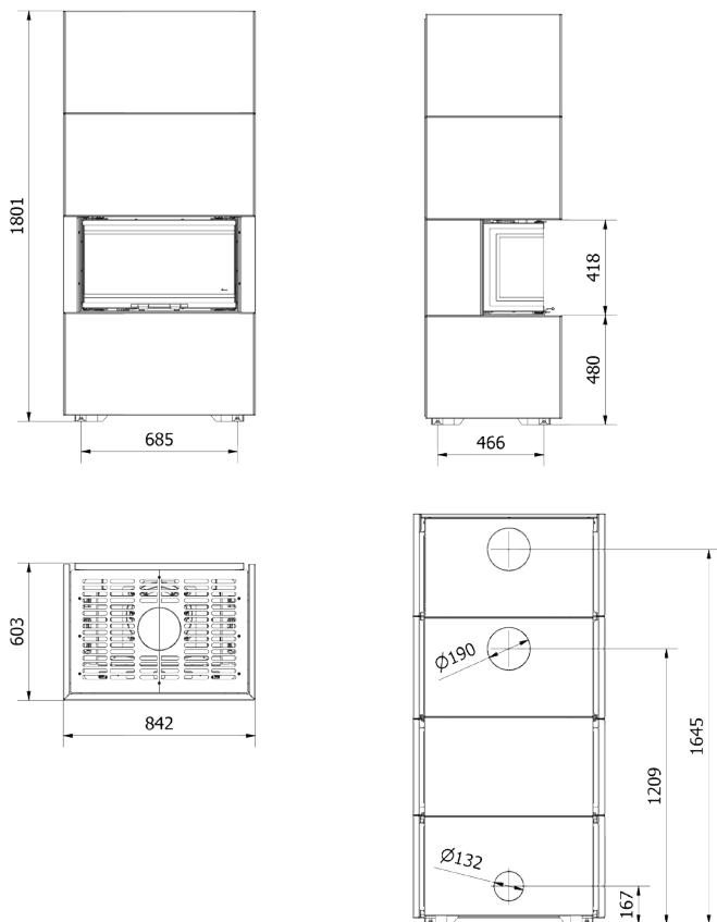
Obr. 1. Rozměrový náčrtek zástavby HOME EASY BOX
