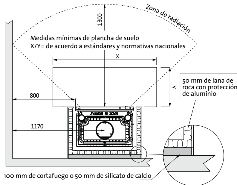
Medidas según EN 13229
