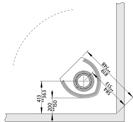
** Jøtul F 162 C / F 163 C, jossa puolieristetty savupiippu/suojattu savuputki tulisijaan saakka.
