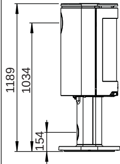
Jøtul F 483 con juego giratorio
