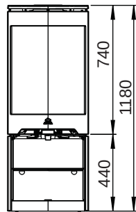
Jøtul F 483 con juego giratorio
