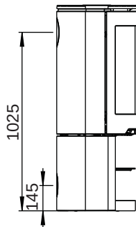
Jøtul F 483 con juego giratorio
