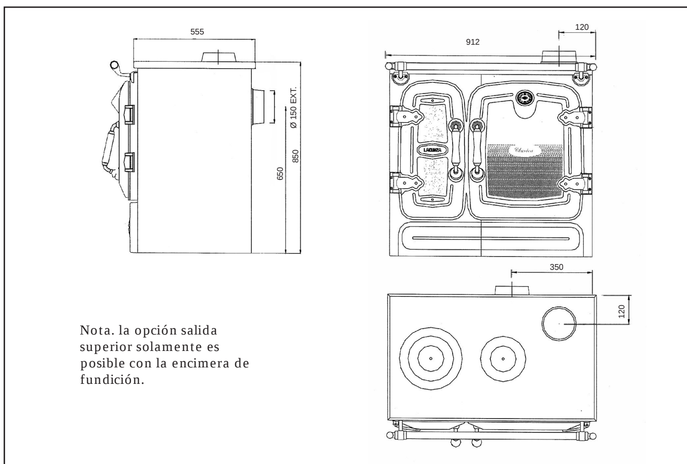
Figura nº 2 - Dimensiones en mm. Cocina Clásica 7.
