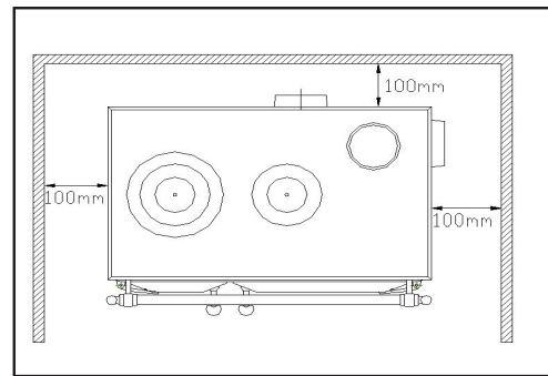
Figura nº4 - Separación mínima de instalación
