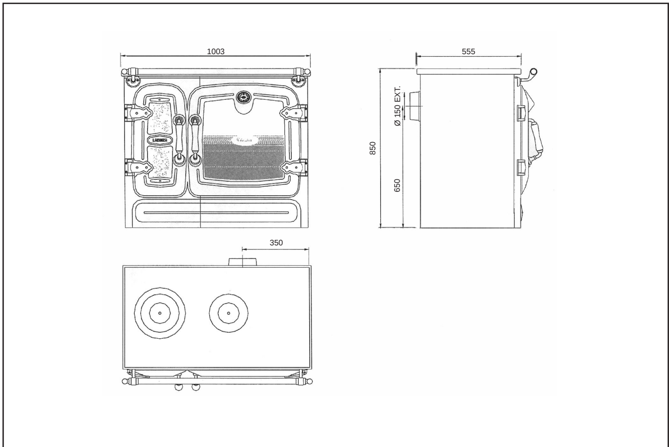
Figura nº 3 - Dimensiones en mm. Cocina Clásica 8.
