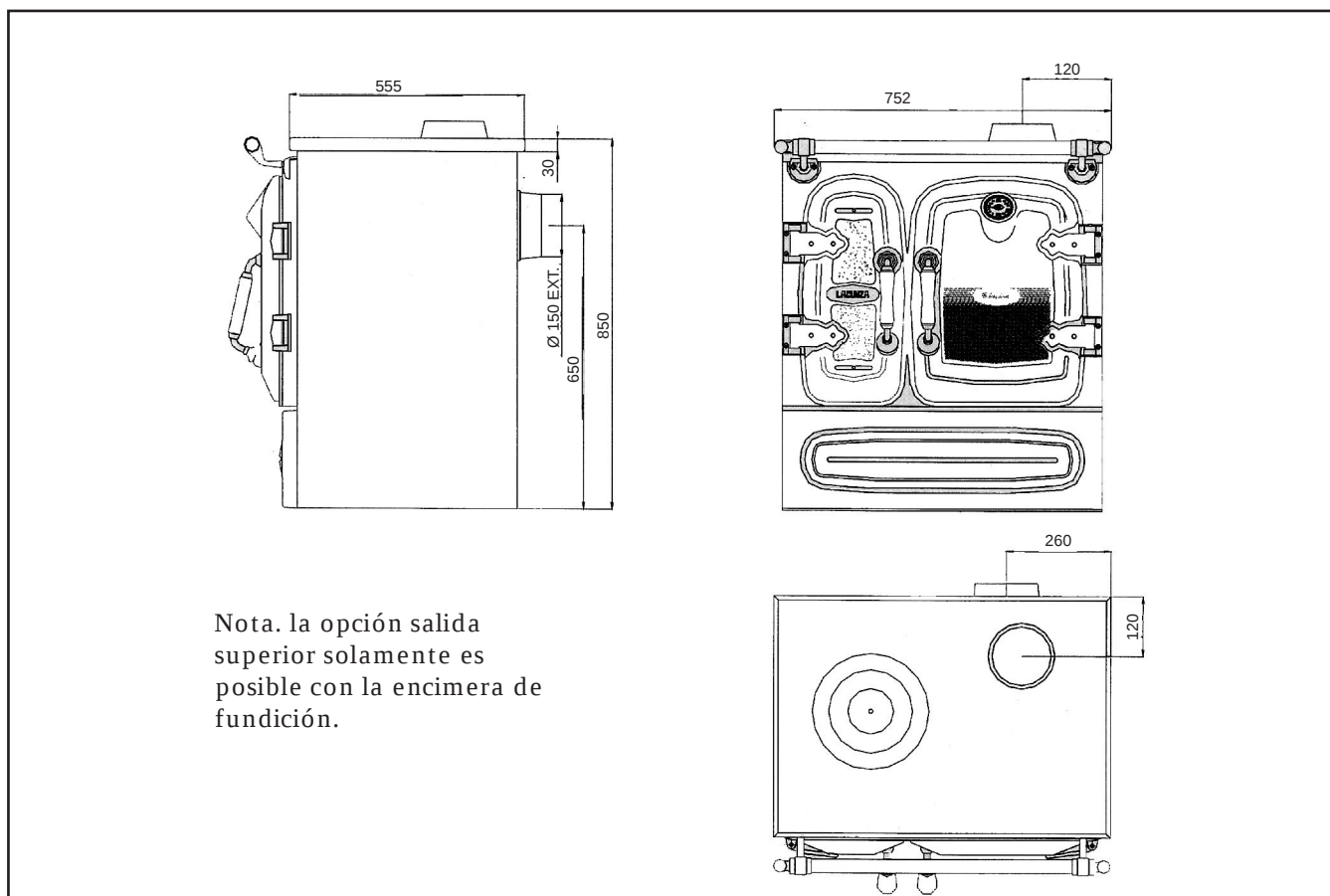
Figura nº 1 - Dimensiones en mm. Cocina Clásica 5.
