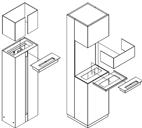
Rys. 6. Montaż biokominka: a) Romeo, b) Sierra, c) Galina
