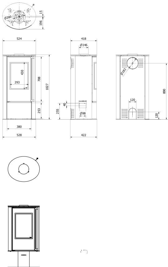
73. Zwymiarowany rysunek pieca ERIK / Dimensioned Figure of the ERIK / Maßzeichnung des Ofens ERIK / Рисунок камина ERIK с определением размеров.
