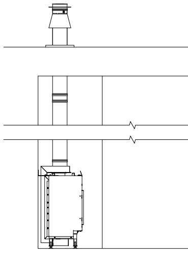
Rys. 9. Wyprowadzenia koncentrycznego systemu kominowego przez dach
