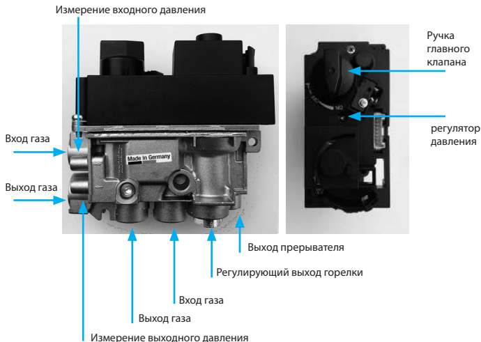
Рис. 20. Регулятор GV60 в базовом положении
