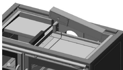
Sistema para acceso al sellado y limpieza de la chimenea
